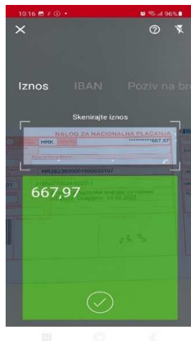
Slika 16 - Djelomično skeniranje
