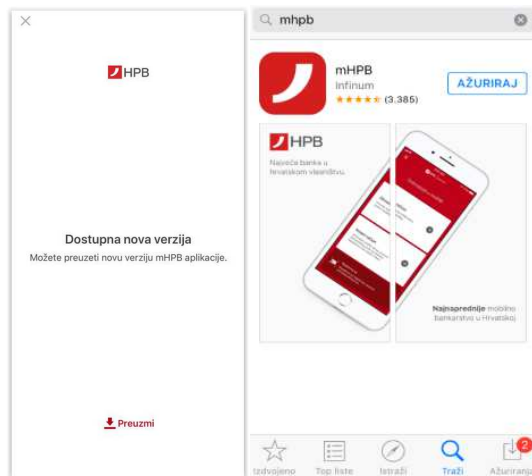
Slika 7 – Nadogradnja aplikacije
