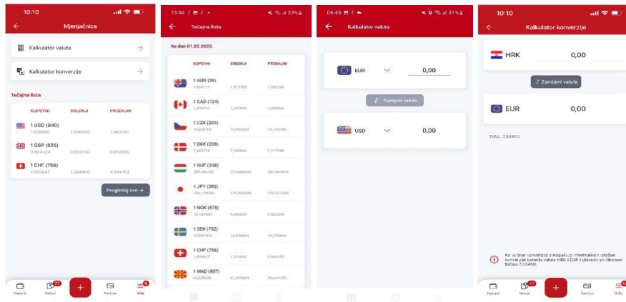
Slika 41 - Mjenjačnica
