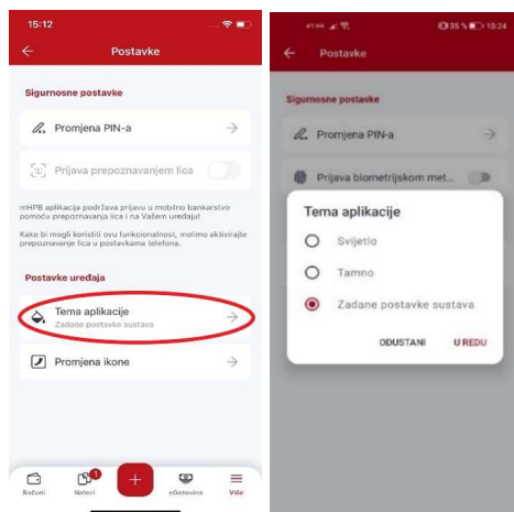
Slika 36 - Tema aplikacije
