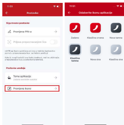
Slika 37 - Promjena ikone
