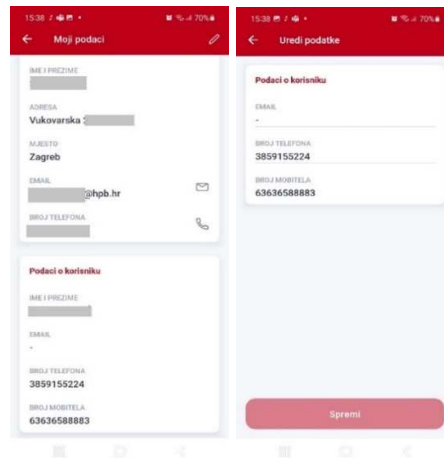
Slika 30- Moji podaci
