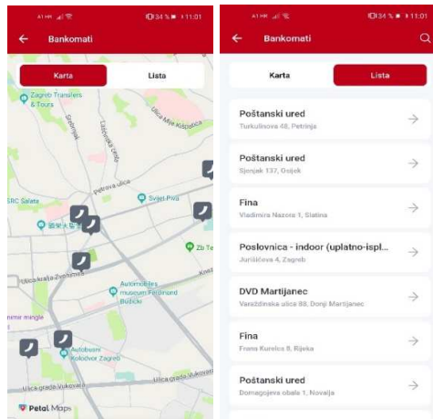
Slika 39 - Bankomati
