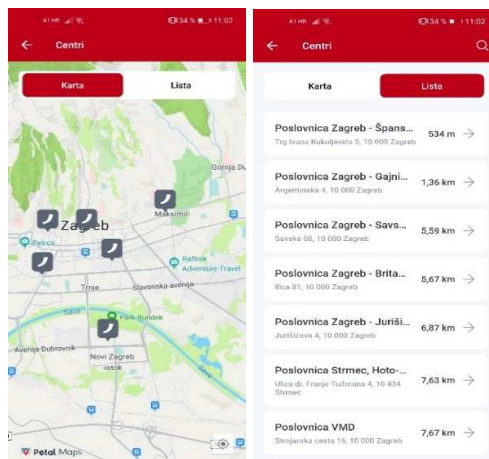
Slika 40 - Centri
