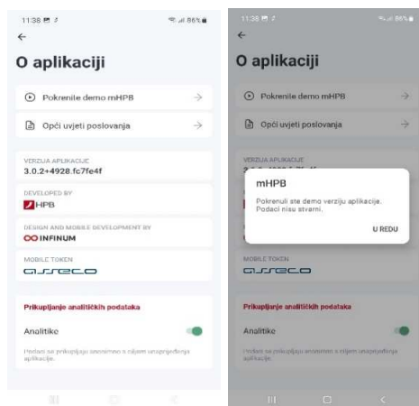
Slika 43 - O aplikaciji
