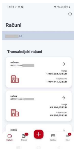
Slika 9 – Moji računi
